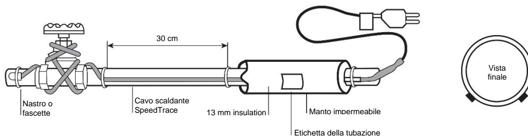
Figura 2 Installazione instradamento a spirale
