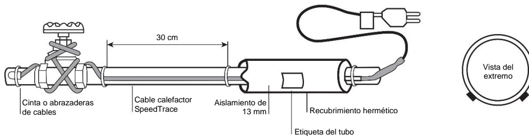
Figura 2 Instalación de trazado a espiral
