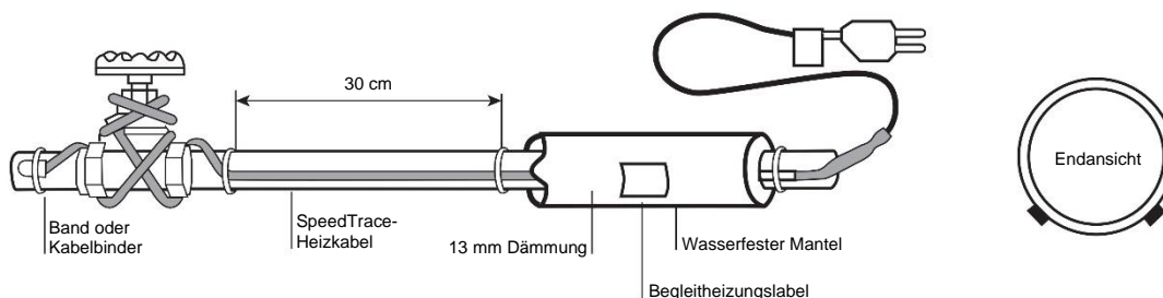
Abbildung 2: Installation in Spiralverlauf
