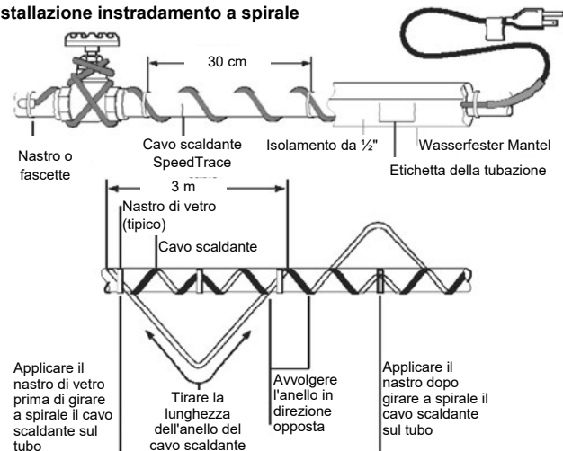
Figura 2 Installazione in strada a spirale
